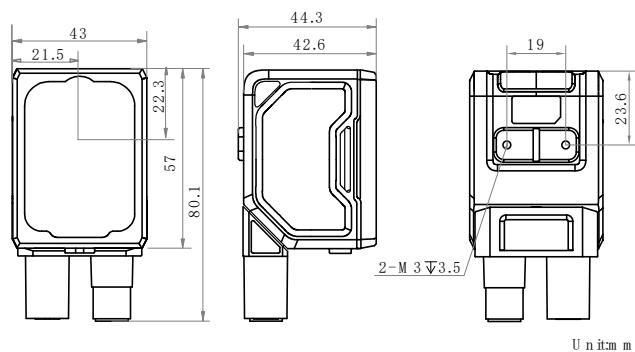
设备 (平角):
