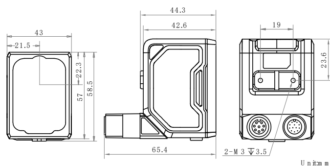
设备（直角）：
